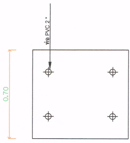
แบบขยายฝาท่อระบายน้ำ ขนาดจริง
