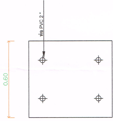
แบบขยายฝาท่อระบายน้ำ ขนาดจริง
